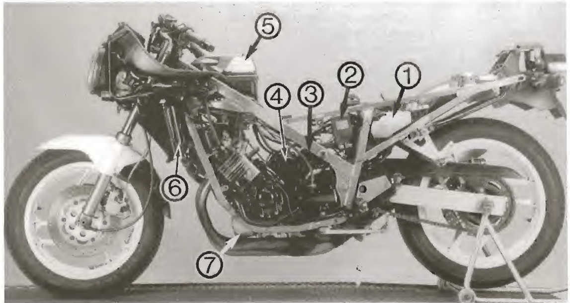
Bild 2 Seitenansicht von links 1 Kühlmittel-Ausgleichsbehälter 2 Zündbox 3 Starter 4 Generator 5 Luffilter 6 Kühler 7 Ölfilter
