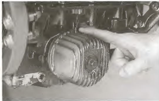
Bild 36 Ölfiltergehäuse. Schlitz muss in Nut eingreifen
