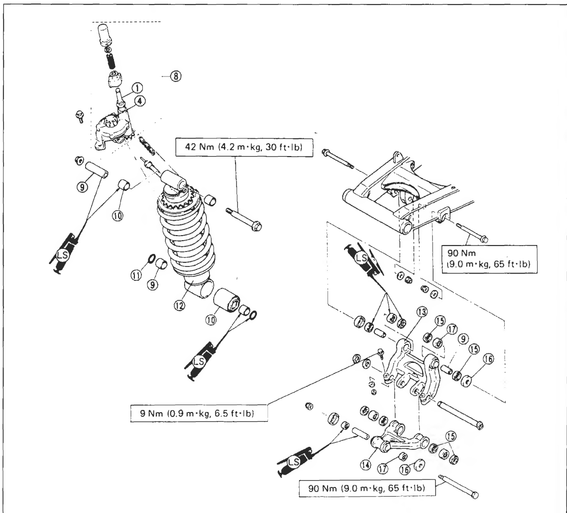
Bild 173 Stossdämpfer und Federbauteile der ersten Ausführung 1 Vorspannungs-Einsteller 4 Dämpfungseinsteller 8 Fernbedienungseinheit 9 Hülse 10 Buchse 11 O-Ring 12 Federbein 13 Verbindungsarm 14 Pleuelstange 15 Dichtring 16 Druckdeckel 17 Lager LS-Fett
