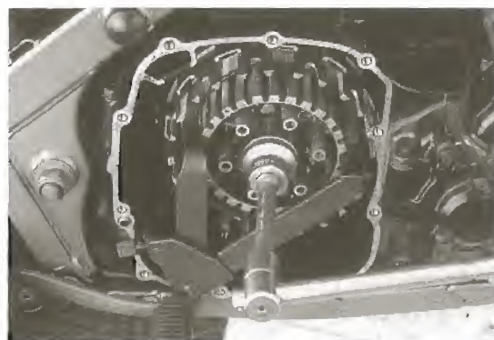
Bild 88 Kupplungshalter ansetzen und Mutter aus- / eindrehen
