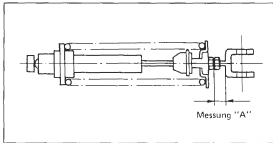
Bild 54 Federvorspannung einstellen
