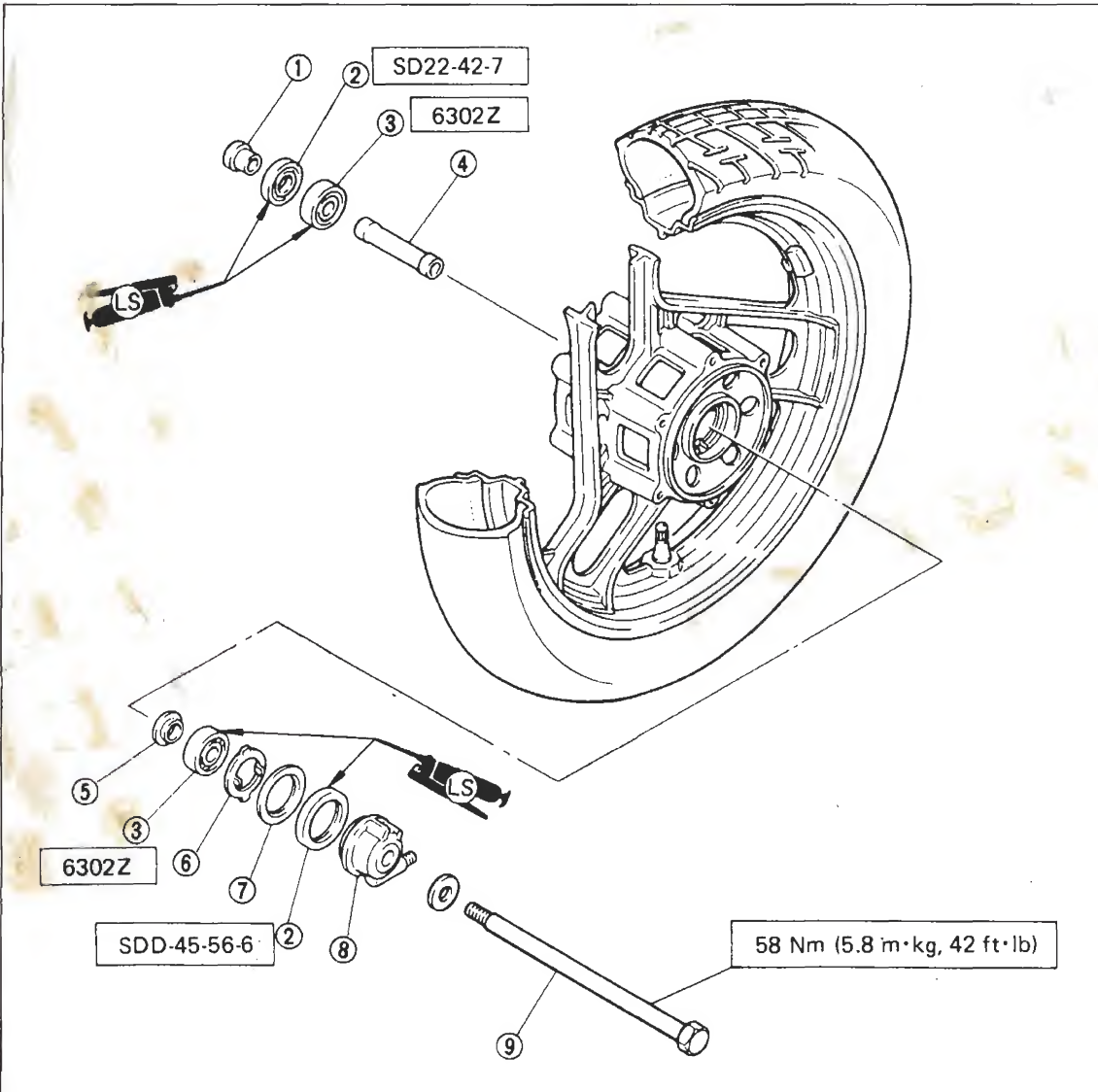
Bild 169 Vorderrad 1 Distanzstück 2 Dichting 3 Lager 4 Distanzhülse 5 Distanzring 6 Tachomitnehmer 7 Halter 8 Tachoschnecke 9 Achse LS-Fett
