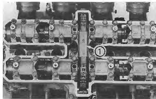
Bild 23 Nockenwellen­lagerdeckel 1 Steuerkettengleitschiene
