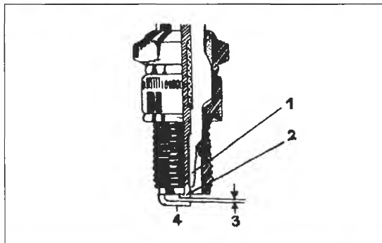
Bild 30 Zündkerze 1 Isolierkörper 2 Mittelelektrode 3 Elektrodenabstand 4 Masselektrode
